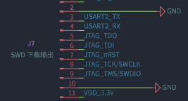
SWD/JTAG 输出
